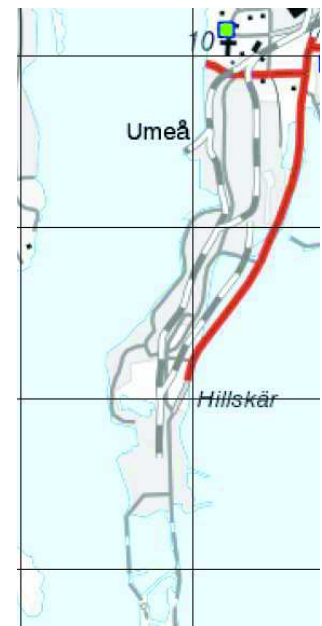
Figur 8. Grundvatten och brunnar. © Sveriges geologiska undersökning.
